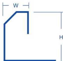
施工示意圖
